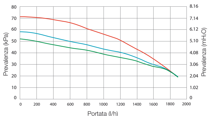
Grafico portata e prevalenza EOLO Superior 32 kW Plus
