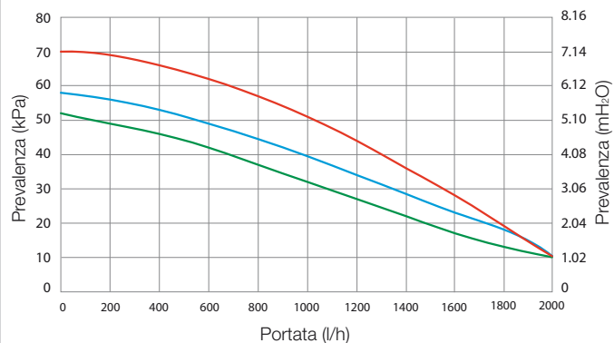
Grafico portata e prevalenza ZEUS Superior 32 kW
