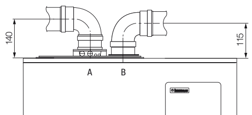
Quota kit separatore Ø 80/80
