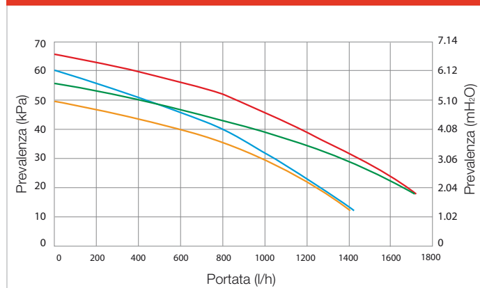
Grafico portata e prevalenza EXTRA Intra 32 kW X
