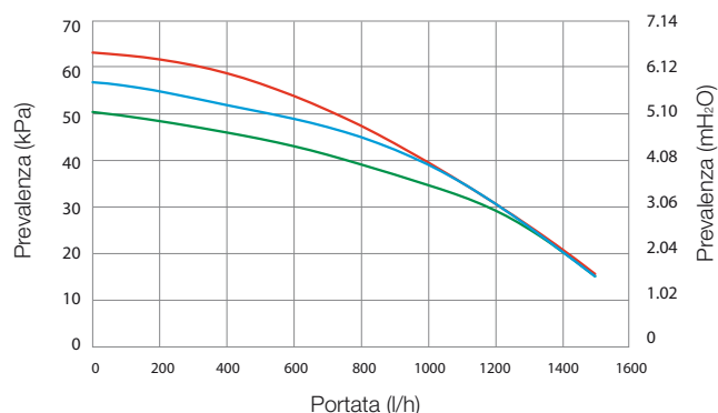
Grafico portata e prevalenza EOLO Eco 28 kW
