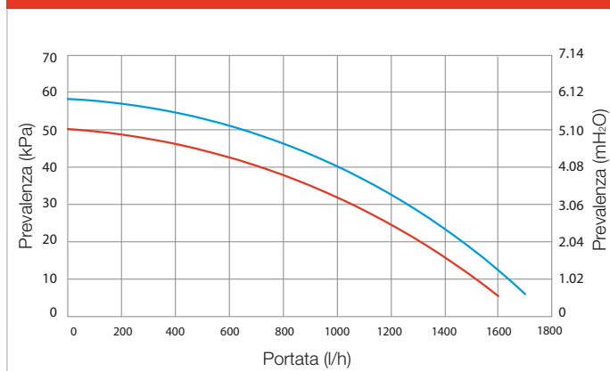
Grafico portata e prevalenza EOLO Extra 24/28 kW
