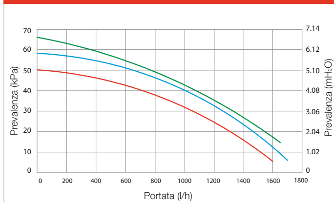
Grafico portata e prevalenza EXTRA Intra 24/28/32 kW
