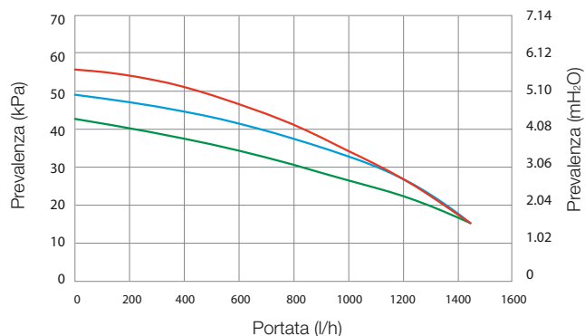
Grafico portata e prevalenza ZEUS Superior 32 kW
