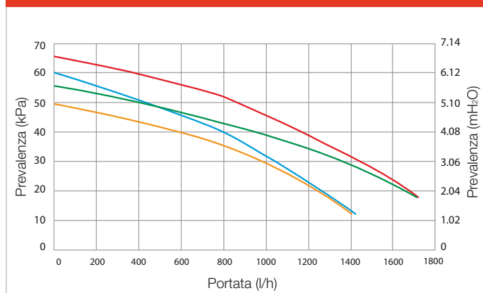
Grafico portata e prevalenza EOLO Extra 32 kW X
