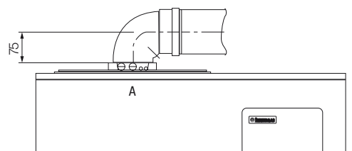
Quota kit concentrico Ø 60/100
