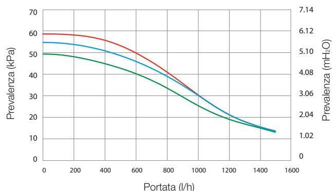
Grafico portata e prevalenza EOLO Eco 24 kW
