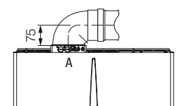
Quota kit concentrico Ø 60/100
