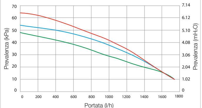
Grafico portata e prevalenza ZEUS Superior 28 kW
