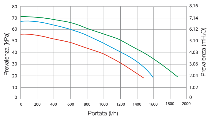
Grafico portata e prevalenza EOLO Superior 24/28/32 kW
